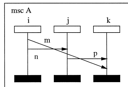
Fig. 2. Example MSC.
