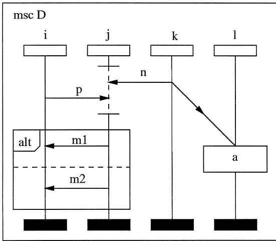
Fig. 5. Example MSC D .
